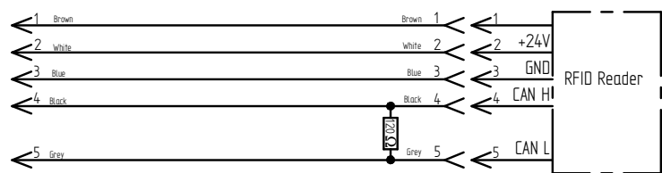
Display RFID Reader
